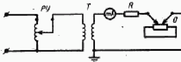
PV—регулирующее устройство; T—трансформатор; R—сопротивление 0,5 МОм; O—образец из карболита с нанесенной пленкой испытуемой эмали.
